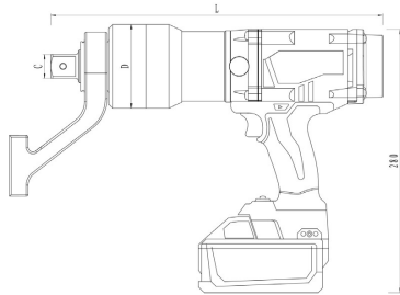
RMW充电扭矩扳手尺寸示意图
